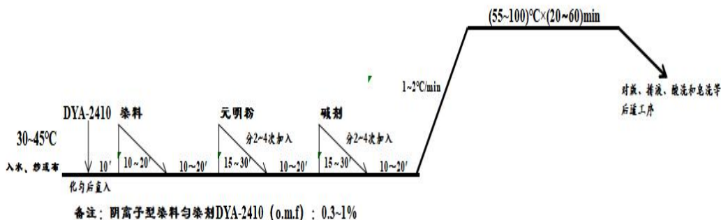
染色工艺流程示意图
